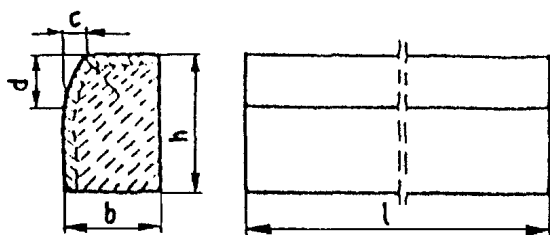
Rys. 1. Wymiarowanie krawężników
